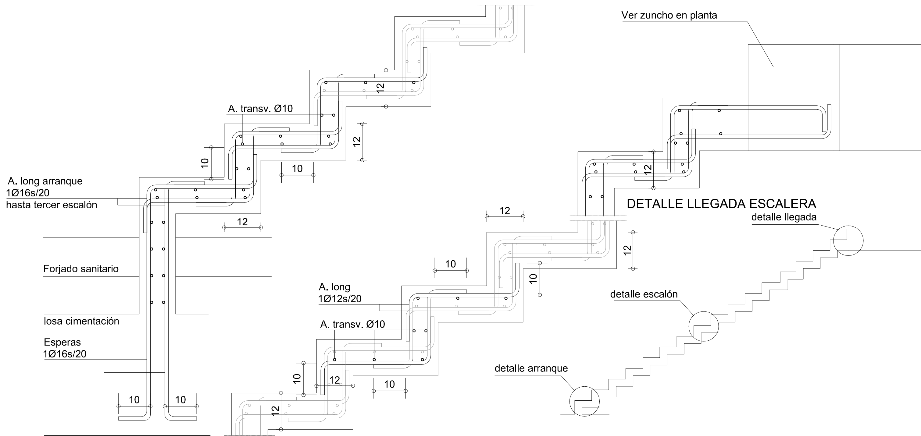
DETALLE ARRANQUE ESCALERA DIN-A1 - Esc. 1/10
