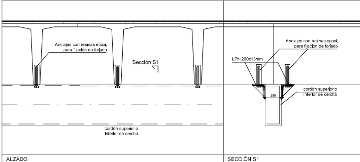
DETALLE 2 esc. 1/20
