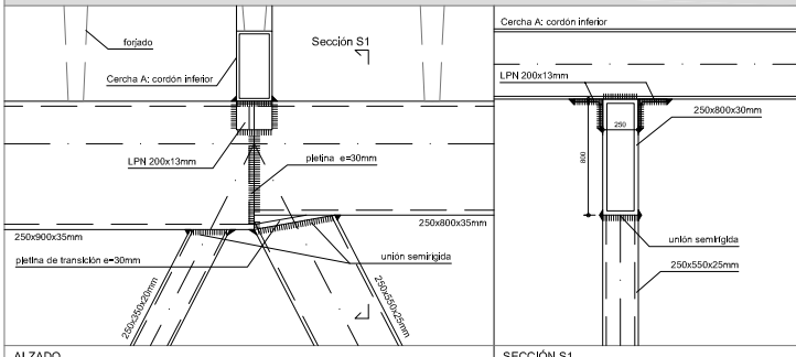
DETALLE 3 esc. 1/20
