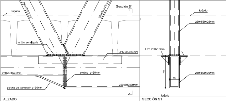
DETALLE 5 esc. 1/20
