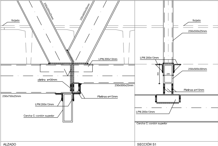
DETALLE 5 esc. 1/20
