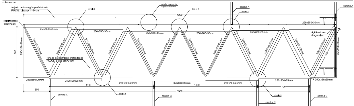
DETALLE 1 - APOYO DE FORJADO EN CORDONES DE CERCHA esc. 1/20
