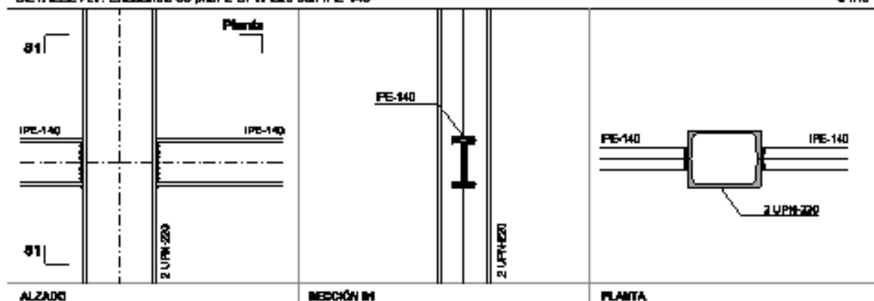
DETALLE A.7: Encuentro de pilar 2 UPN-220 con IPE-140
