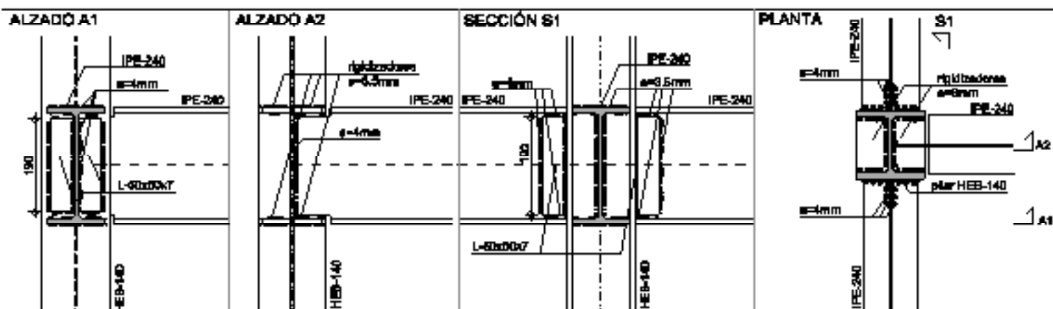
DETALLE DE UNIÓN DE PILAR HEB-140 CON VIGA IPE-240
