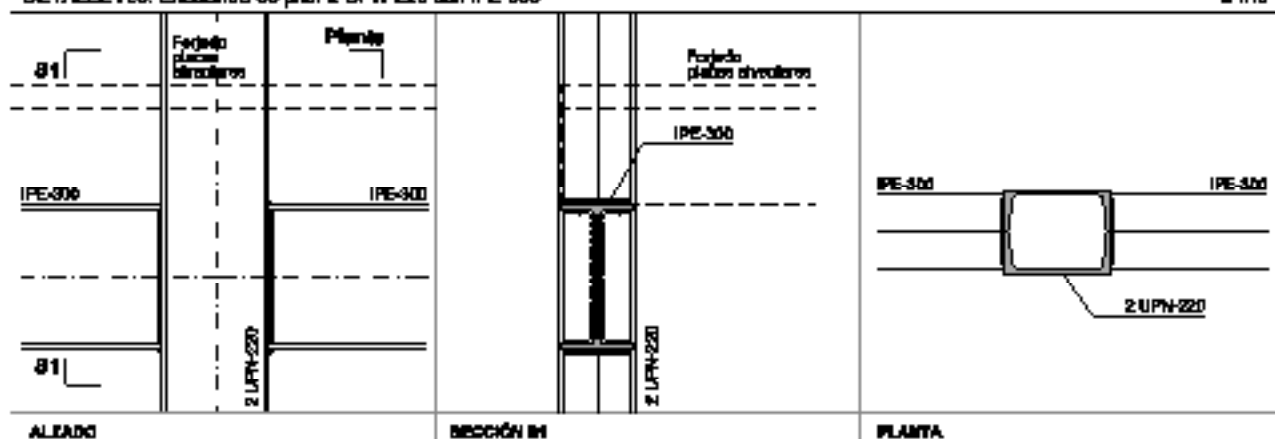
DETALLE A.8: Encuentro de pilar 2 UPN-220 con IPE-300
