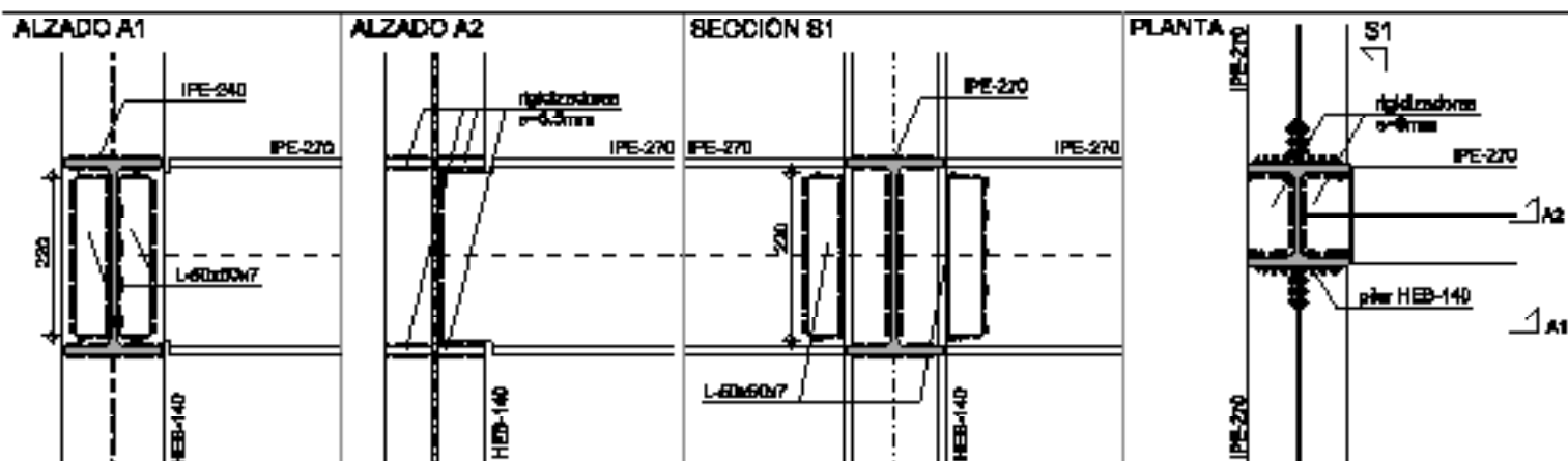
DETALLE DE UNIÓN DE PILAR HEB-140 CON VIGA IPE-270
