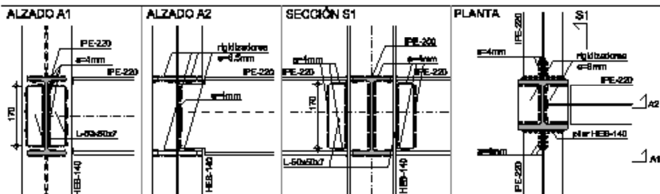
DETALLE DE UNIÓN DE PILAR HEB-140 CON VIGA IPE-220
