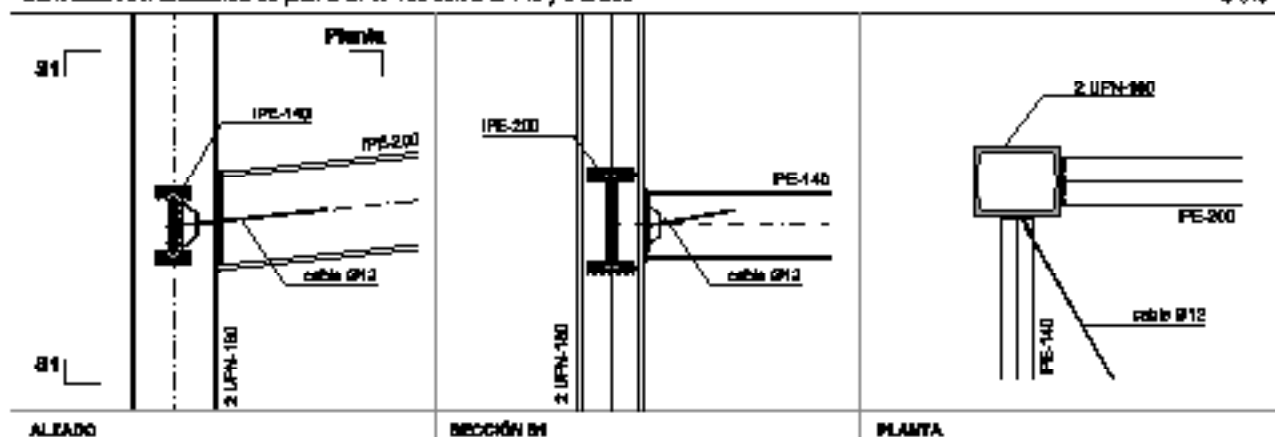
DETALLE A.1: Encuentro de pilar 2 UPN-160 con IPE-140 y IPE-200
