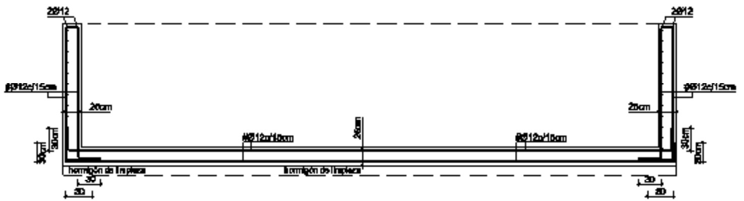
DETALLE PISCINA SECCIÓN S1
