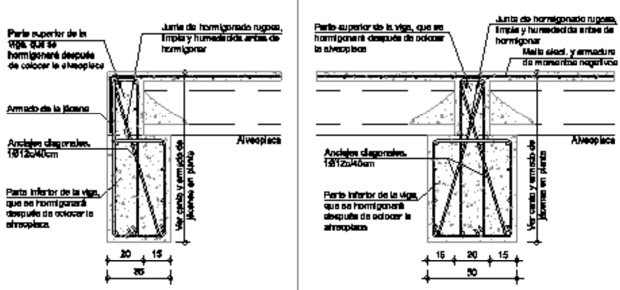
DETALLE DE FORJADO DE PLACAS ALV. EN JÁCENAS DE CANTO DE H.A. esc. 1/20
