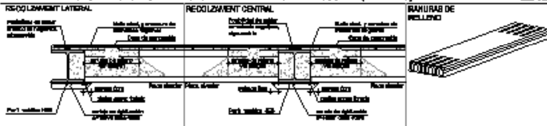
DETALLE DE APOYO DE FORJADO DE PLACAS ALV. EN PERFILES METÁLICOS HEB (EMBEBIDO) Ese. 1/20
