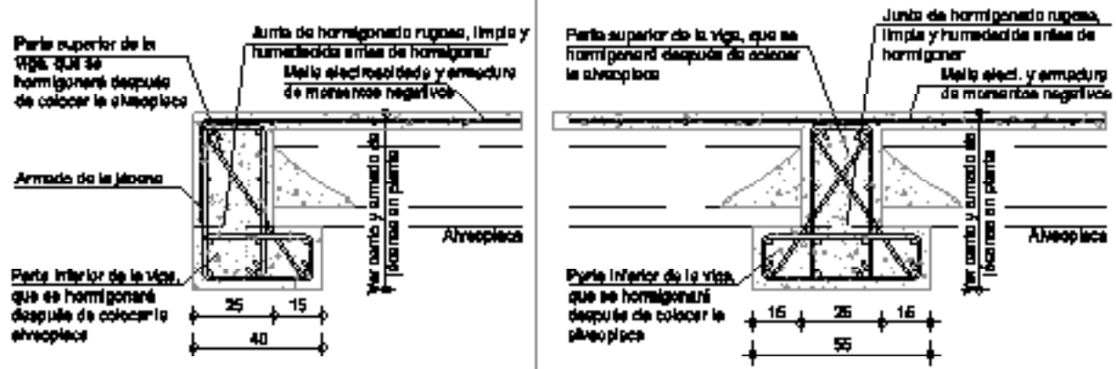
DETALLE DE FORJADO DE PLACAS ALV. EN JÁCENAS DE CANTO DE H.A. esc. 1/20
