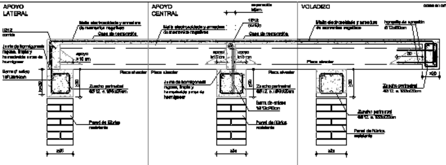
DETALLE DE APOYO DE FORJADO DE PLACAS ALV. EN PARED DE FÁBRICA RESISTENTE
