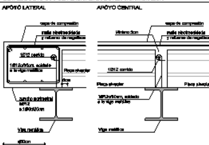
DETALLE DE APOYO DE PLACA ALVEOLAR EN VIGA METÁLICA Ese. 1/10
